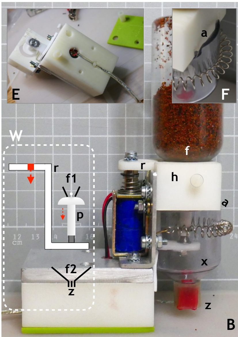
Fish feeder (design). Øyvind Teig, Trondheim. 9.2019
