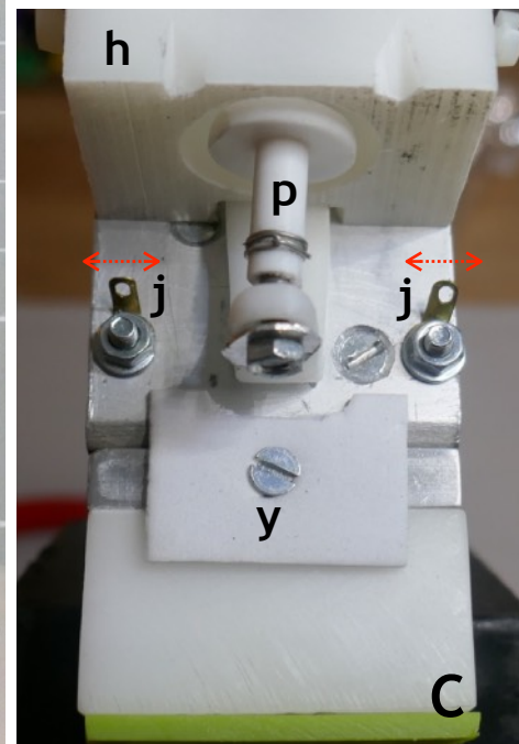
Fish feeder (design). Øyvind Teig, Trondheim. 9.2019
